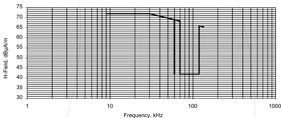
Figuur 3: 9-135 kHz, magnetisch veld limieten op 10 meter meetafstand
